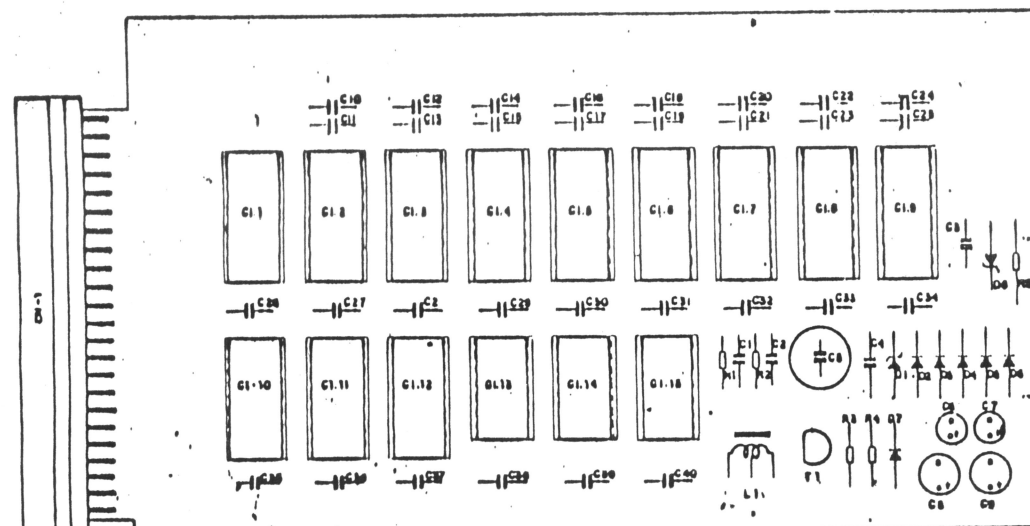
PLANTA
