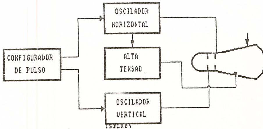
- PCI DEFLEXÃO - DIAGRAMA EM BLOCOS
