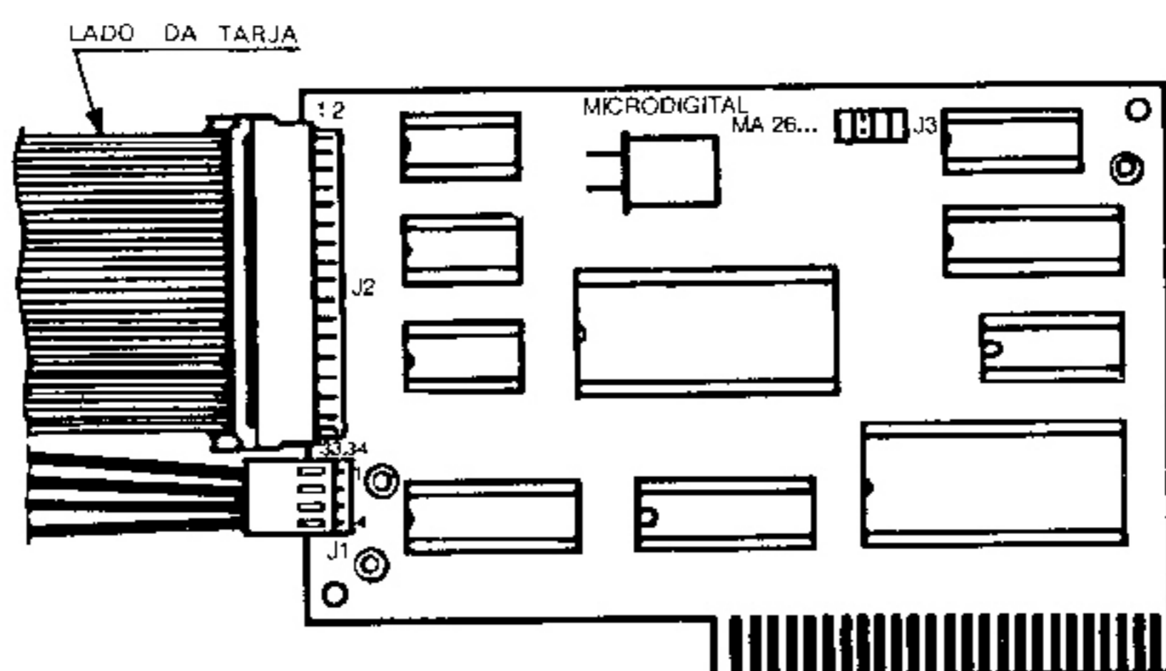
FIGURA 1 – Conexão dos cabos na placa
